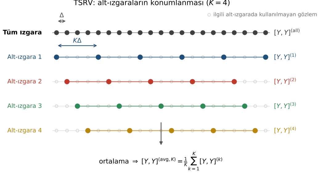
Şekil 6: TSRV’de alt-ızgaraların konumlanması ( M = 21 gözlem, K = 4 ). En üstte tüm-ızgara: ardışık gözlemler \Delta aralıklıdır ve [Y, Y]^{(all)} bu ızgaradan hesaplanır. Altındaki dört satır alt-ızgaraları gösterir: k ’nci alt-ızgara k, k + K, k + 2K, \dots indeksli gözlemleri alır; içi dolu noktalar o alt-ızgarada kullanılan, içi boş halkalar kullanılmayan gözlemlerdir. Her alt-ızgarada ardışık gözlemler arası aralık K\Delta ’dır — yani her biri seyrek örneklenmiş bir seridir. Alt-ızgaralar örtüşmez ve birlikte tüm veriyi tüketir; bu nedenle K tahmin ortalandığında veri kaybı olmaz.
